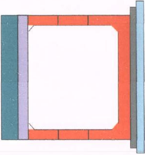
BOX CULVERT 16+600
